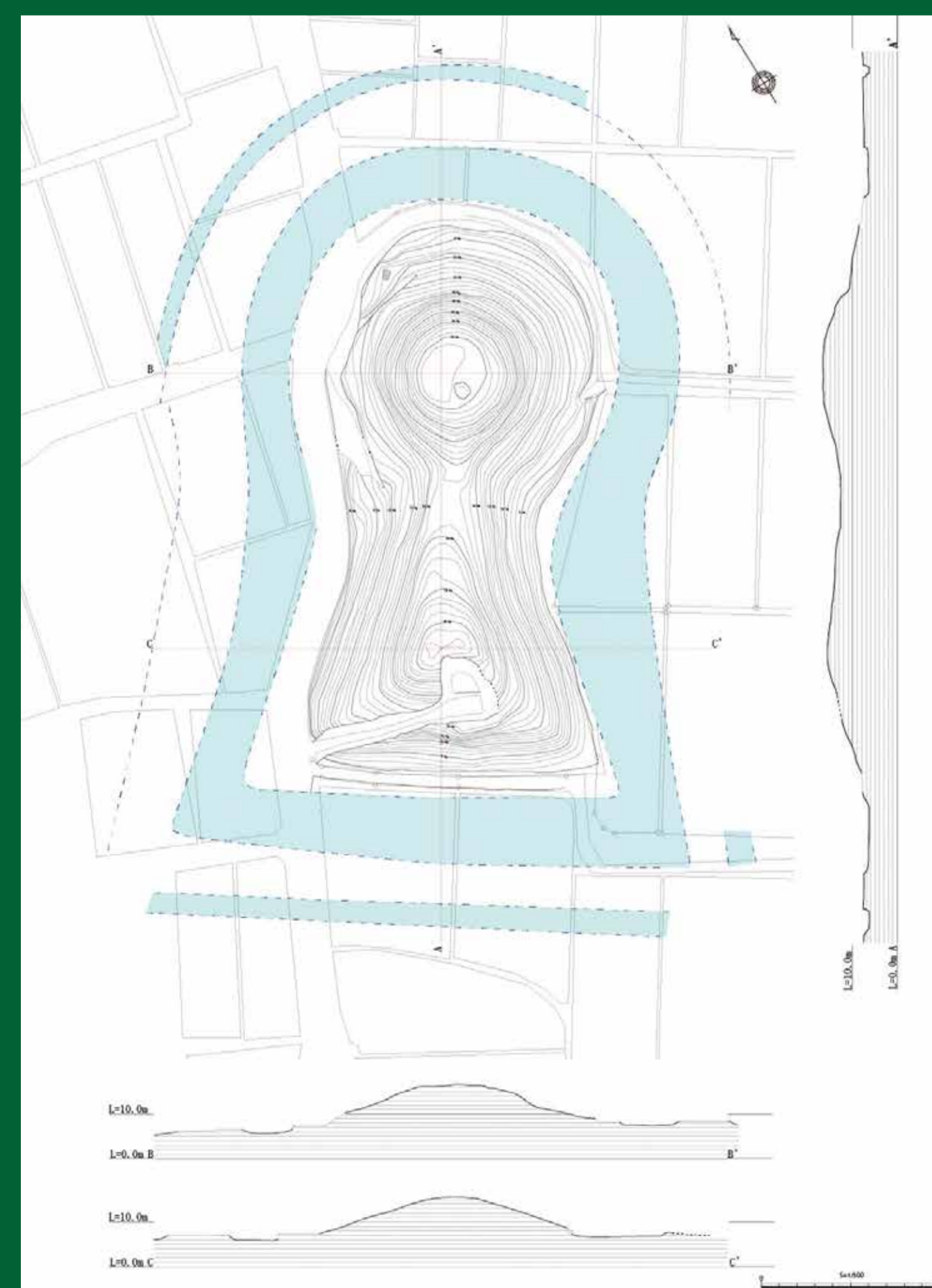
【測量平面断面図】
